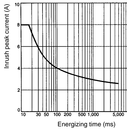
G3MC-101P(L), G3MC-201P(L)
