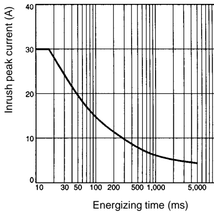
G3MC-202P(L)
